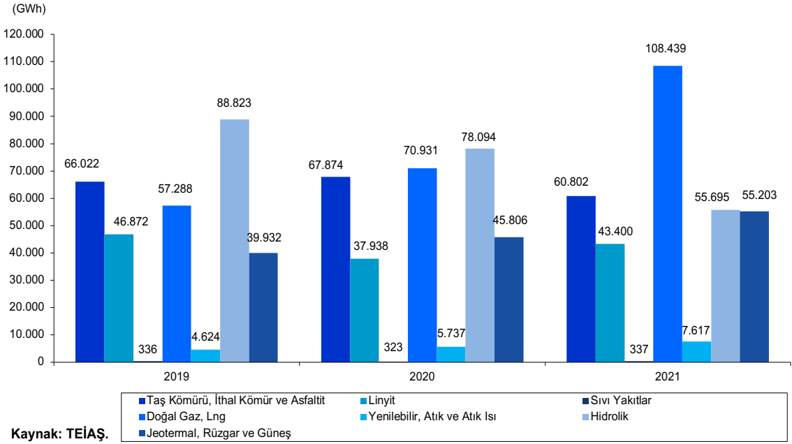
Grafik 16. Elektrik Enerjisi Üretiminin Birincil Enerji Kaynaklarına Göre Dağılımı
